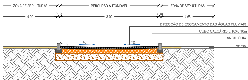
PORMENOR P02
