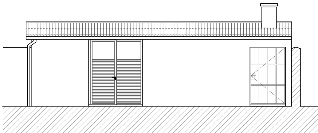
Alçado Principal
