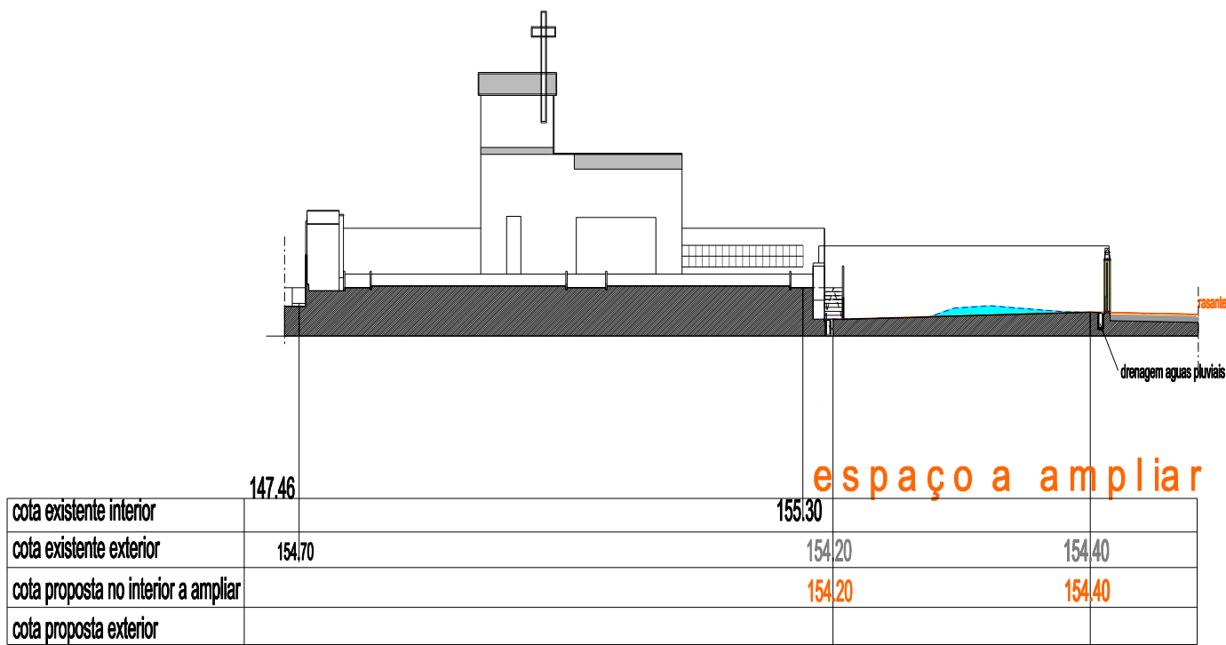
Perfil transversal 1
